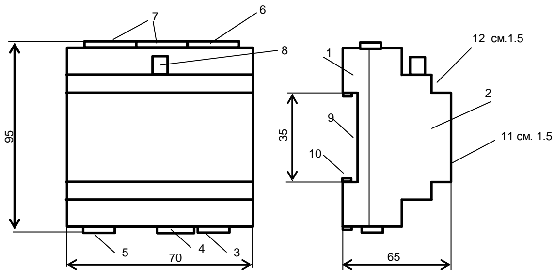
Рисунок 3 – габаритные и установочные размеры модема
