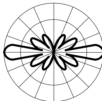
Рисунок 2 - диаграмма направленности антенны в вертикальной плоскости
