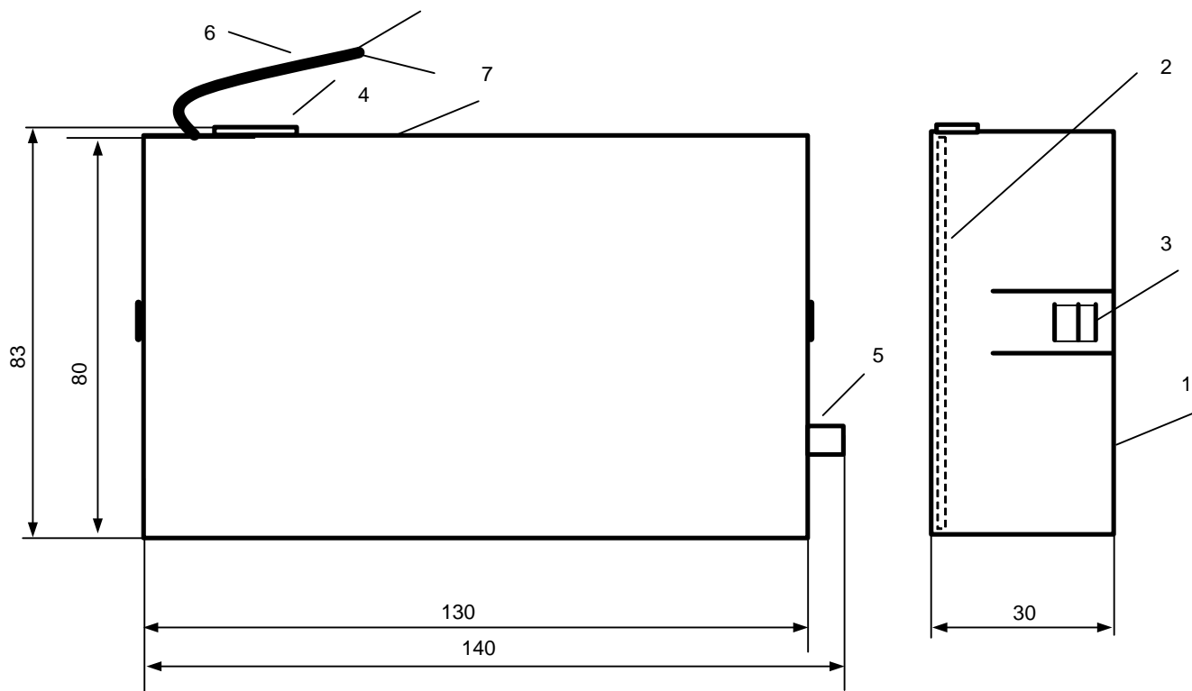
Рисунок 2 - габаритные размеры модема
