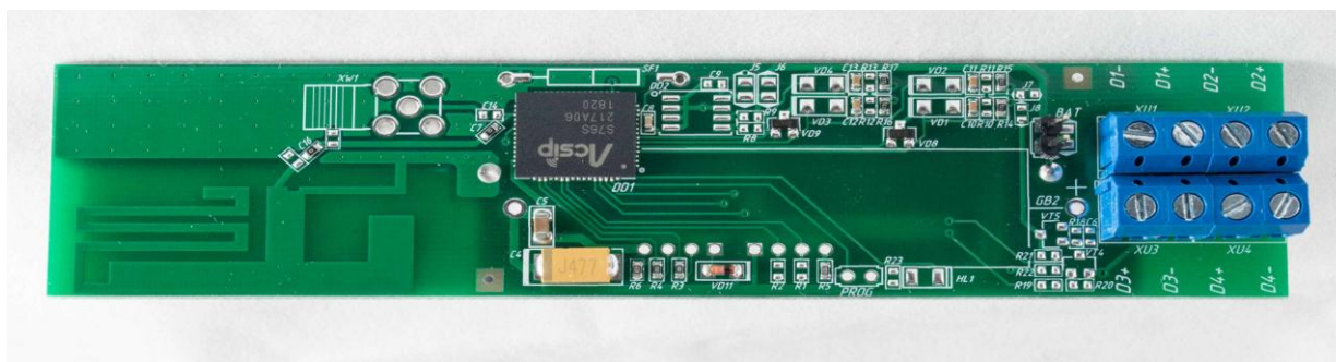
Рисунок 4 - контакты принудительной передачи, исполнение «в тубе»
