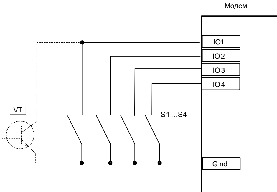
Рисунок Г.1 - схема подключения выходов датчиков к дискретным входам, модем МУР 1001.9 GSM/GPRS TLT Н1-Н2-IO4-Н4-Н5-Н6, S1...S4 – «сухой контакт», VT – открытый коллектор
