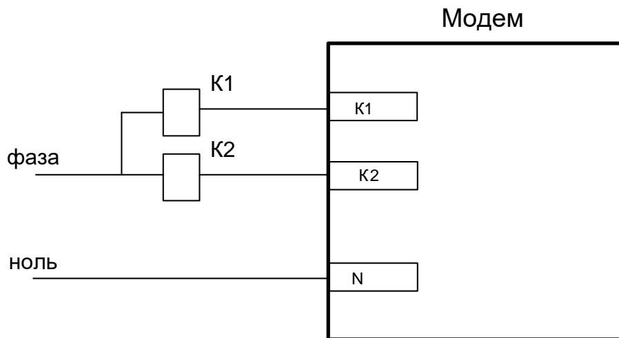
Рисунок Г.2 - схема подключения нагрузки (реле K1 и K2) к сети 230 В, модем МУР 1001.9 GSM/GPRS TLT Н1 - SWR – Н3-Н4-Н5-Н6
