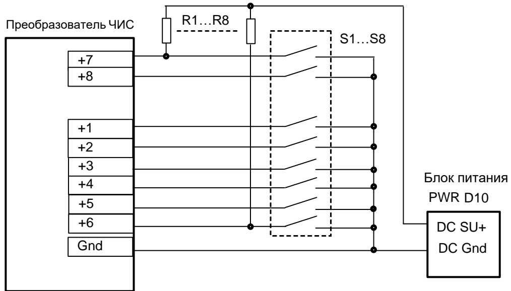
Рисунок В.1 - вариант исполнения преобразователя ЧИС МУР 1001.5 ADN- PE-H2-H3,
