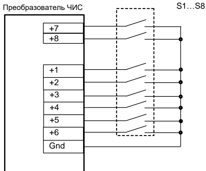
Рисунок В.2 - вариант исполнения преобразователя ЧИС МУР 1001.5 ADN-PW-H2-H3,
