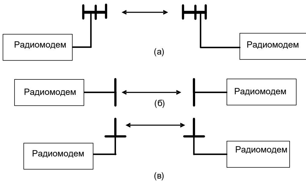
Рисунок 2 - правильное расположение антенн радиомодемов в пространстве: (а) – направленные антенны: логопериодические, волновые каналы, (б) - антенны типа « диполь», (в) - штыревые антенны
