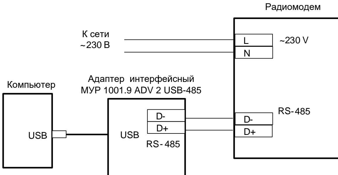
Рисунок Б.2 - интерфейсы связи RS-485 - радиомодема и USB - компьютера
