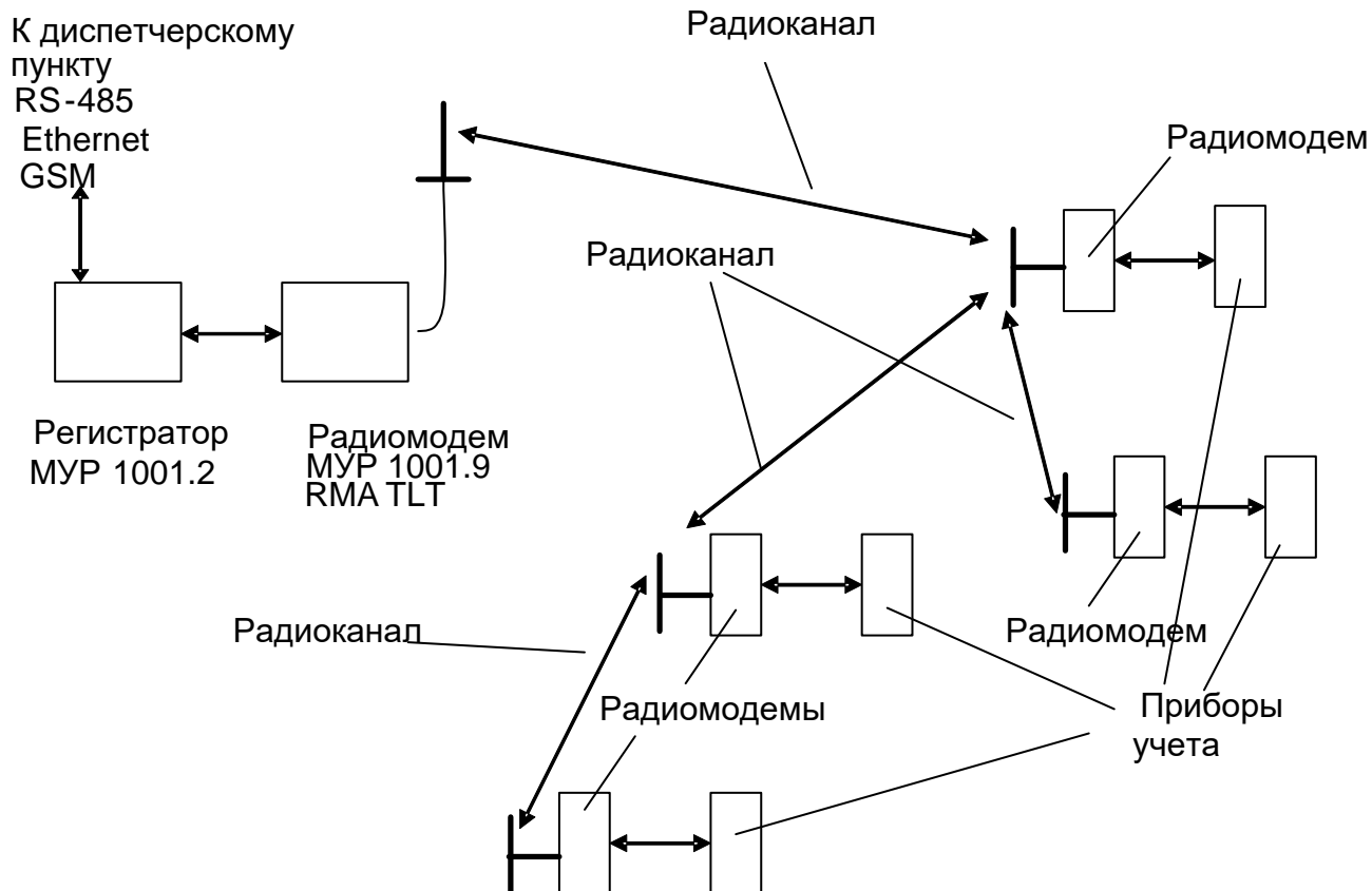
Рисунок 1 - пример схемы построения элемента информационно-измерительного комплекса МУР 1001 с использованием радиомодемов
