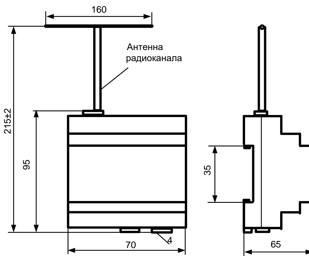
Рисунок 3. габаритные и установочные размеры радиомодема
