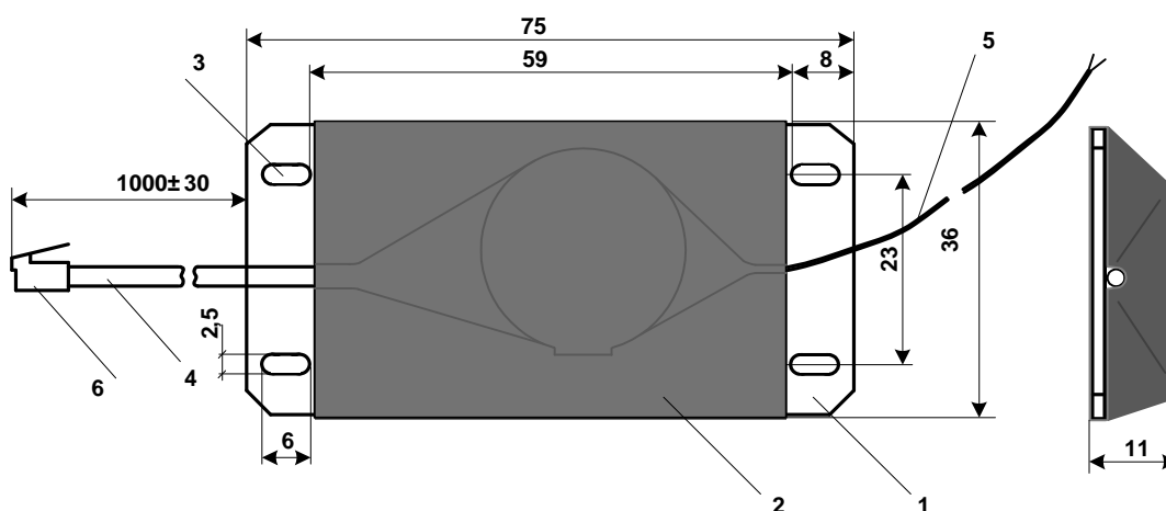
Рисунок 2 - габаритные и установочные размеры преобразователя ЧИС
